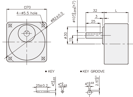
K7G□B(C)
